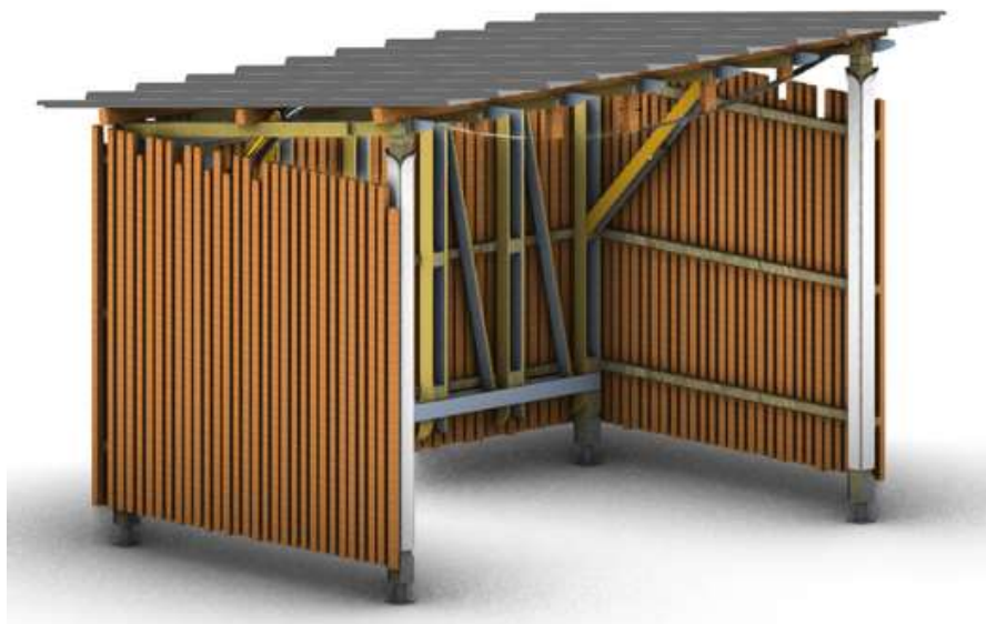
Vue en 3D d'un abri à vélos avec un bardage en bois
